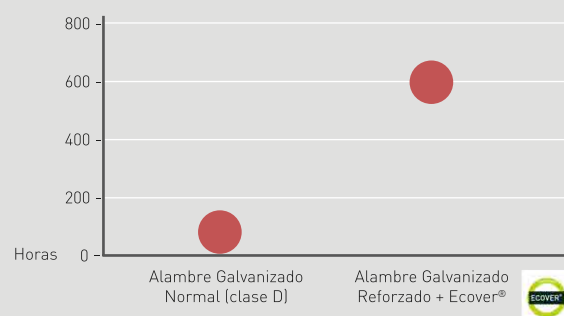
Inicio de la corrosión roja en Cámara de Niebla Salina Ensayo de corrosión roja en atmósferas artificiales según la Norma ISO 9227
